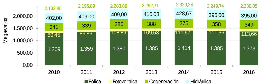
Potencia de energía instalada (en funcionamiento) procedente de fuentes renovables en la provincia de Zaragoza
