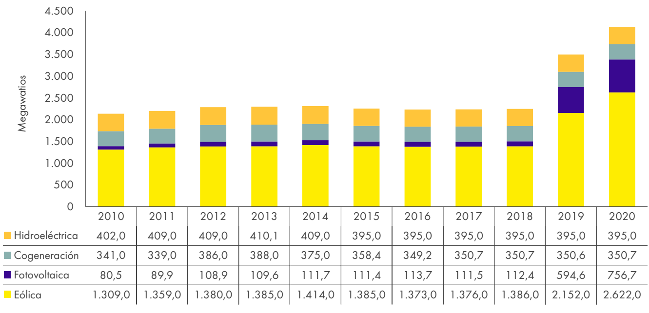
Evolución de la potencia de energía instalada (en funcionamiento) procedente de fuentes renovables en Zaragoza provincia, 2010-2020
