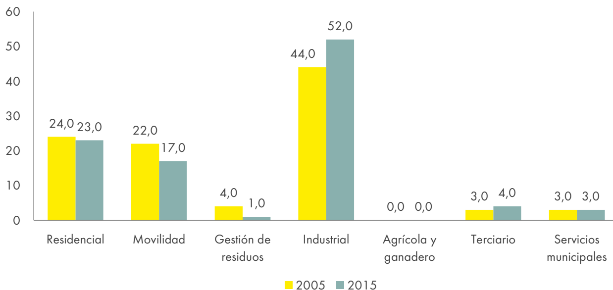
Origen de las emisiones de CO 2 por sectores en la ciudad de Zaragoza (%), 2005-2015
