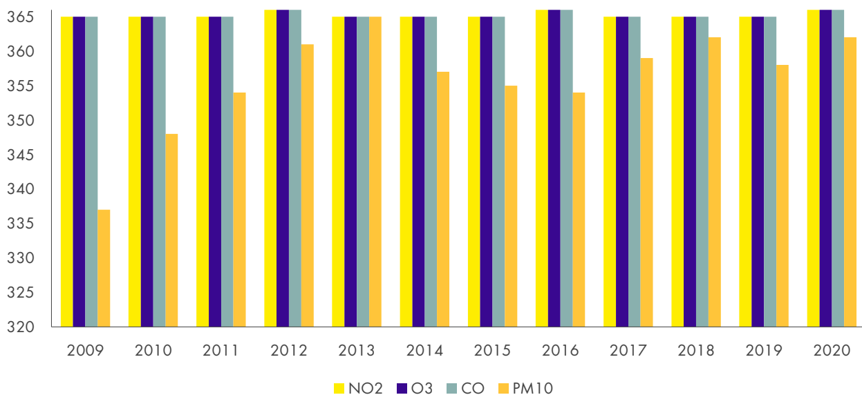
Evolución del número de días con buena calidad de aire en la ciudad de Zaragoza, 2009-2020
