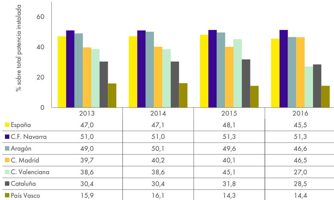
Evolución de la potencia eléctrica instalada con fuentes renovables, 2013-2016
