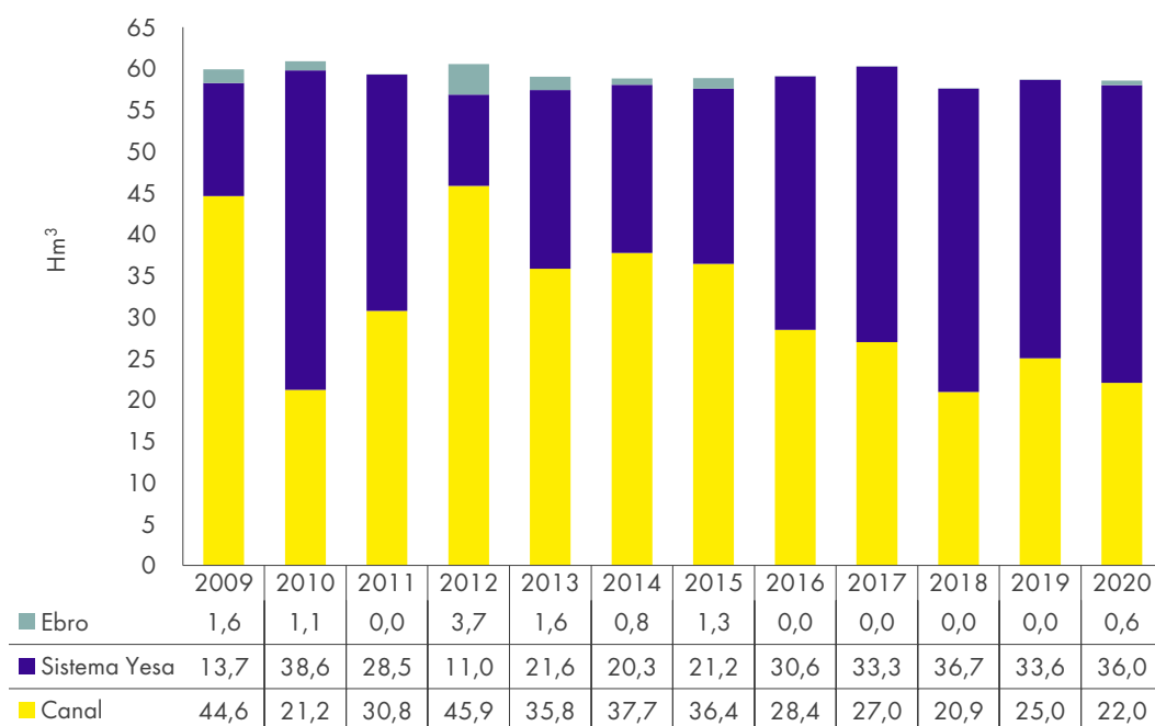
Evolución de la captación total de agua, 2009-2020
