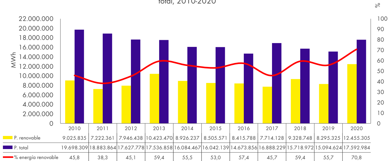
Evolución de la producción energética en Aragón y porcentaje de energía renovable respecto al total, 2010-2020
